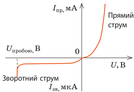
Вольт-амперна характеристика (ВАХ) напівпровідникового діода
