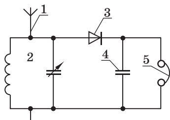
Рис. 23.9. Електрична схема найпростішого радіоприймача:
