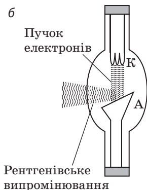
Рис. 35.3. Рентгенівська трубка: а — вигляд; б — схематичне зображення
