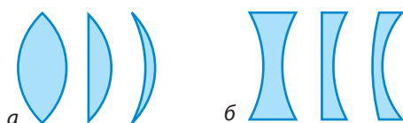
Рис. 27.1. Різні види лінз у розрізі: а — опуклі лінзи (двоопукла, плоско-опукла, увігнуто-опукла); б — увігнуті лінзи (двоввігнута, плоско-ввігнута, опукло-ввігнута)
