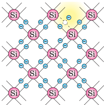
Рис. 9.3. Схематичне зображення ковалентного зв'язку кремнію
