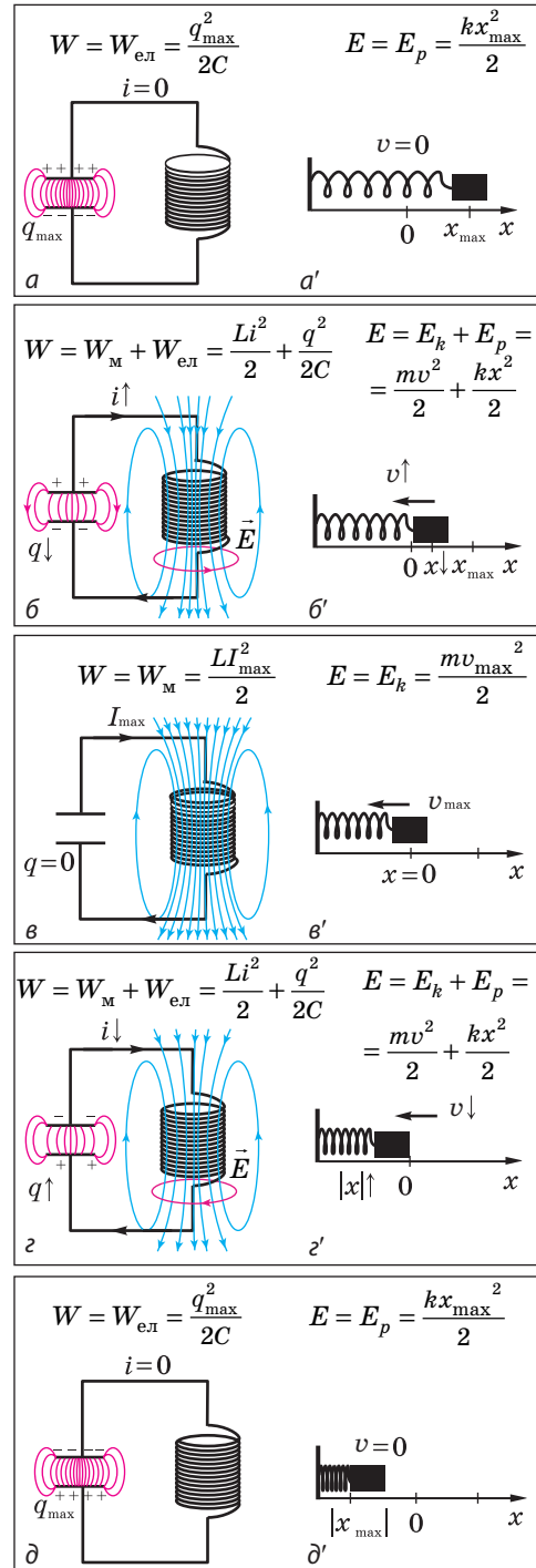
Рис. 18.2. Механізм вільних електромагнітних коливань у коливальному контурі (а–д) і механізм вільних механічних коливань тягарця на пружині (а'–д')
