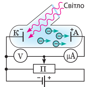
Рис. 34.2. Схема дослідів для вивчення фотоефекту
