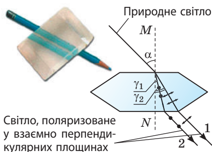
Рис. 32.3. Подвійне променезаломлення природного світла в монокрystalі ісландського шпату. MN — оптична вісь кристала (світло, напрямлене вздовж оптичної осі, не заломлюється і не роздовжується)
