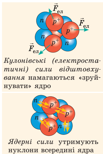
Рис. 39.3. Сили взаємодії між нуклонами всередині ядра
