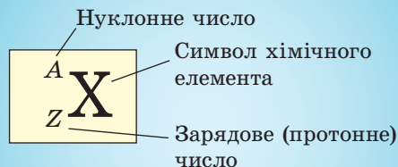
Рис. 39.1. Позначення нукліда хімічного елемента
