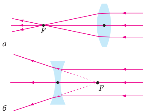
Рис. 27.3. Хід променів у лінзах: а — збиральна лінза, точка F — головний дійсний фокус лінзи; б — розсіювальна лінза, точка F — головний уявний фокус лінзи
