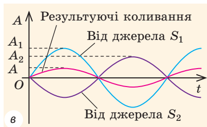
Рис. 30.1. Якщо хвилі надійшли в точку M (а) в однаковій фазі, амплітуда результатуючих коливань збільшується: A = A_1 + A_2 (б), а якщо хвилі надійшли в протилежних фазах, амплітуда результатуючих коливань зменшується: A = A_1 - A_2 (в)
