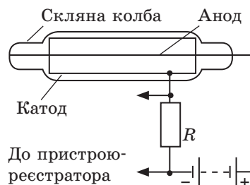
Рис. 41.6. Будова газорозрядного лічильника (лічильника Гейгера — Мюллера)
