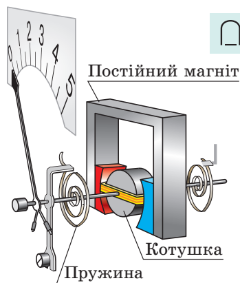
Вимірювальний механізм приладів магнітоелектричної системи
