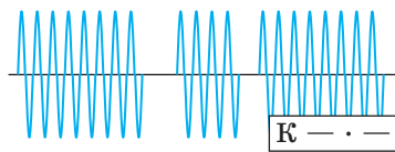
Рис. 23.3. Радіотелеграфний сигнал є низкою короточасних і більш тривалих імпульсів електромагнітних хвиль
