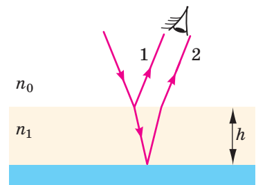
Рис. 30.3. Розділення пучка світла на два когерентні пучки на тонкій прозорій плівці; n_0 — показник заломлення повітря, n_1 — показник заломлення плівки, h — товщина плівки
