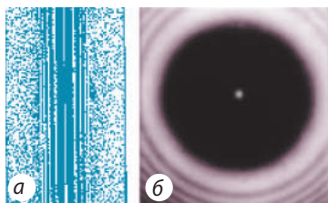
Рис. 31.2. Дифракція світлових хвиль на різних перешкодах: на тонкому дроті (а); на великому непрозорому круглomu екрані (б)
