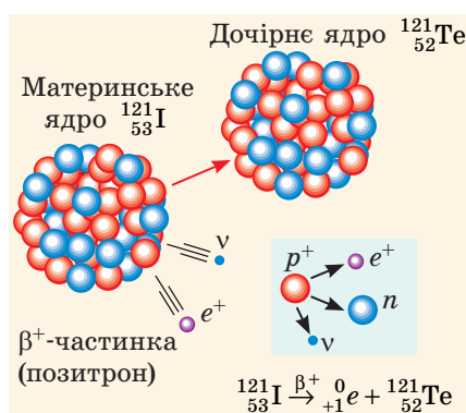
Рис. 40.4. Під час \beta^+ -розпаду один із протонів материнського ядра перетворюється на нейтрон, позитрон й електронне нейтрино: {}_1^1p \rightarrow {}_0^1n + {}_{+1}^0e + {}_0^0v ; позитрон і нейтрино випромінюються, нейтрон залишається в ядрі (утворюється нове ядро)
