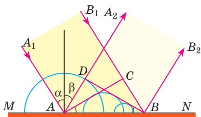
Рис. 25.6. Відбивання плоскої хвилі від плоскої поверхні MN : хвильова поверхня падаючої хвилі — площа AC , відбитої хвилі — площа DB ; \alpha — кут падіння, \beta — кут відбивання
