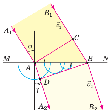
Рис. 26.2. Заломлення плоскої хвилі на плоскій межі поділу MN : хвильова поверхня падаючої хвилі — площа AC , заломленої хвилі — площа DB ; \alpha — кут падіння, \gamma — кут заломлення
