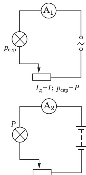
Рис. 20.2. До введення поняття «діюче значення сили струму»
