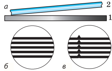
Рис. 30.6. Перевірка якості шліфування за допомогою інтерференції. Якщо зразок (1) гладенький, то інтерференційні смуги паралельні (б); якщо ж на поверхні зразка є подрипини — інтерференційні смуги викривлені в бік збільшення товщини повітряного клину (в)
