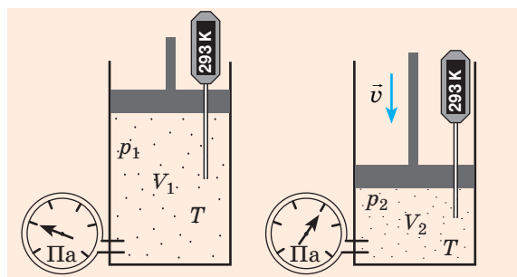
Рис. 30.2. Ізотермічне стисання газу. Якщо повільно опускати поршень, температура газу під поршнем буде лишатися незмінною і дорівнюватиме температурі навколишнього середовища. Тиск газу при цьому буде збільшуватися
