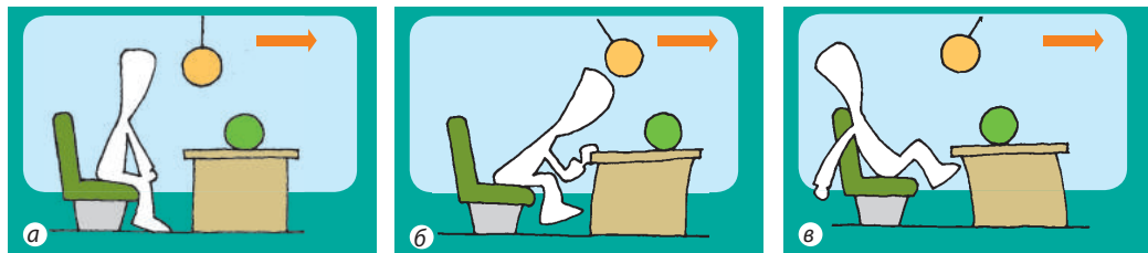
Рис. 9.3. СВ, пов'язана з потягом, буде інерціальною, тільки коли потяг відносно Землі перебуває в стані спокою або рухається рівномірно прямолінійно (а); в усіх інших випадках ця СВ неінерціальна (б, в)
