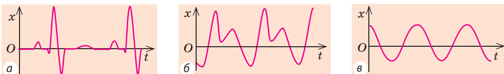
Рис. 19.6. Графіки залежності зміщення x тіла (або частини тіла) від часу t коливань: а — грудна клітина під час серцевих поштовхів (кардіограма); б — мембрана динаміка під час випромінювання звукової хвилі; в — тіло на пружині
