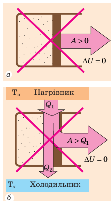
Рис. 38.2. Циклічні процеси, які неможливі з точки зору першого закону термодинаміки
