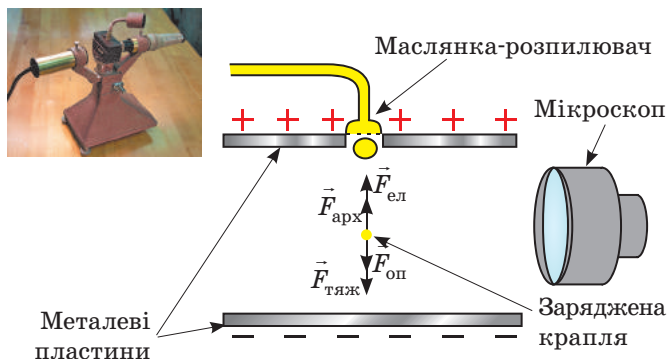
Рис. 40.1. Пристрій для дослідів Р. Міллікена щодо визначення заряду електрона. На краплю, що потрапляє між пластинами, діють сила тяжіння ( \vec{F}_{\text{тяж}} ), сила опору повітря ( \vec{F}_{\text{оп}} ), архімедова сила ( \vec{F}_{\text{арх}} ) і сила з боку електричного поля заряджених пластин ( \vec{F}_{\text{ел}} )
