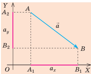
Рис. 3.6. Визначення проєкцій вектора на осі координат: a_x — проєкція вектора \vec{a} на вісь OX , a_x > 0 ; a_y — проєкція вектора \vec{a} на вісь OY , a_y < 0
