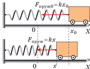
Рис. 16.3. Якщо пружину звільнити, то, стискаючись, вона виконає роботу (надасть руху візку), при цьому деформація пружини зменшиться
