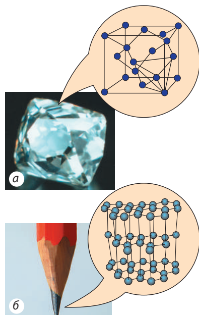
Рис. 34.2. Різні кристалічні стани вуглецю: а — алмаз; б — графіт
