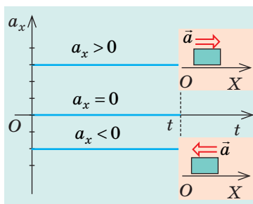
Рис. 6.2. Графік залежності a_x(t) для рівноприскореного прямолінійного руху
