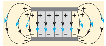
Рис. 41.5. Картина силових ліній електричного поля, створеного системою двох пластин, заряджених рівно за модулем і протилежно за знаком. Синім позначено напрямки векторів напруженості
