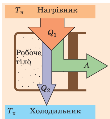
Рис. 39.3. Принцип роботи теплових двигунів: робоче тіло, одержуючи певну кількість теплоти Q_1 від нагрівника, виконує механічну роботу A і передає деяку кількість теплоти Q_2 холодильнику
