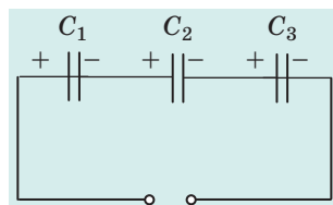
Рис. 44.3. Батарея з трьох послідовно з'єднаних конденсаторів
