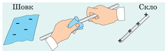
Рис. 40.2. Під час електризації тертям частина електронів зі скляної палички перейде на клатик шовку, в результаті чого скляна паличка набуде позитивного заряду, а клатик шовку — негативного
