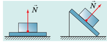
Рис. 12.7. Сила нормальної реакції опори направлена перпендикулярно до поверхні опори
