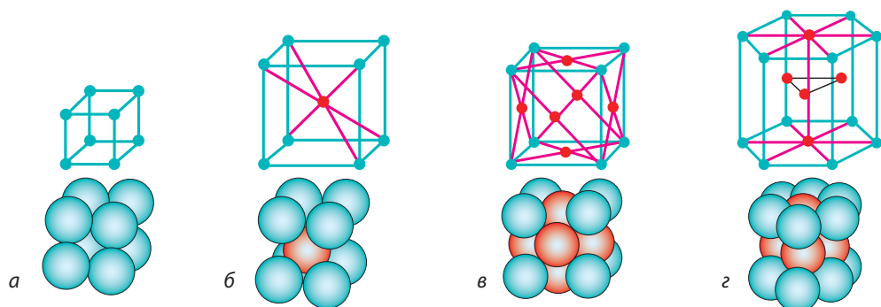
Рис. 34.1. Деякі види кристалічних ґраток: а — проста кубічна; б — об'ємноцентрована кубічна; в — гранецентрована кубічна; г — гексагональна
