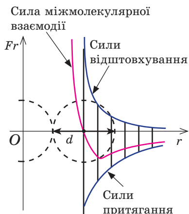
Рис. 27.5. Графіки залежності сил притягання, сил відштовхування та сили міжмолекулярної взаємодії ( F_r ) від відстані r між молекулами. Сила міжмолекулярної взаємодії обчислюється як алгебраїчна сума сил відштовхування та сил притягання
