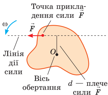
Рис. 14.2. Тіло обертається проти ходу годинникової стрілки відносно осі, що проходить через точку O
