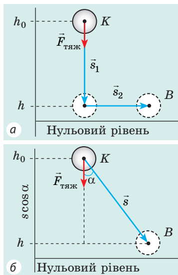
Рис. 16.2. У випадку переміщення тіла з висоти h_0 до висоти h робота сили тяжіння, незалежно від траєкторії руху тіла, визначається за формулою: A = mgh_0 - mgh
