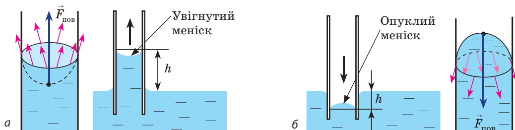
Рис. 33.8. Капілярні явища: а — змочувальна рідина піднімається в капілярі; б — незмочувальна рідина опускається в капілярі
