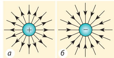
Рис. 41.4. Силові лінії електричного поля, створеного точковим зарядом: a — позитивним; b — негативним
