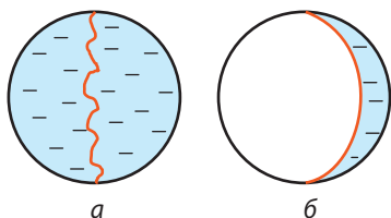
Рис. 33.2. Дослід, що демонструє наявність сил поверхневого натягу
