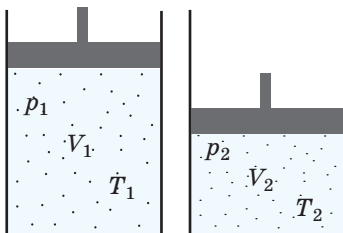
Рис. 30.1. До виведення рівняння Клапейрона
