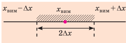
Рис. 2.4. Абсолютна похибка визначає інтервал, у якому перебуває істинне значення вимірюваної величини
