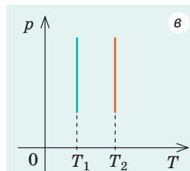
Рис. 30.3. Графіки ізотермічного процесу; T_1 < T_2
