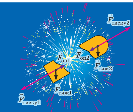
Рис. 17.2. Під час розриву снаряду для феєрверка сумарний імпульс системи зберігається, оскільки в момент розриву зовнішні сили (сила тяжіння та сила опору) незначні порівняно із силами тиску порохових газів
