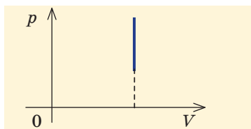
Рис. 37.5. При ізохорному процесі газ роботу не виконує
