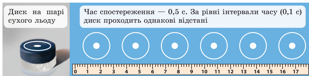
Рис. 9.2. Чим менше тертя (опір рухові тіла), тим більше горизонтальний рух тіла наближається до руху за інерцією
