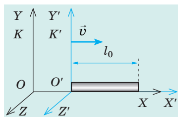
Рис. 25.1. Довжина l стрижня в СВ K , відносно якої стрижень рухається, є меншою від «власної» довжини l_0 стрижня — довжини стрижня в СВ K' , відносно якої стрижень перебуває у спокої
