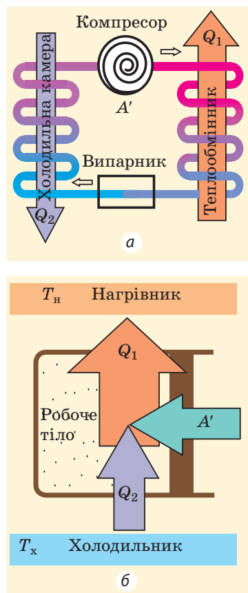
Рис. 39.6. Будова (а) і принцип роботи (б) холодильного пристрою: робоче тіло розширюється і виконує роботу, одержуючи кількість теплоти Q_2 від холодильної камери. За рахунок роботи A' зовнішніх сил робоче тіло стискається, при цьому довкіллю передається кількість теплоти Q_1 = Q_2 + A'
