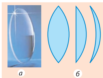
Рис. 14.1. Опукла лінза — лінза, товщина якої посередині більша, ніж біля країв: а — вигляд; б — різні опуклі лінзи в розрізі
