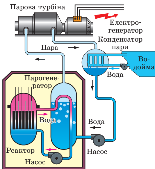
Рис. 26.4. Принцип роботи атомної електростанції
