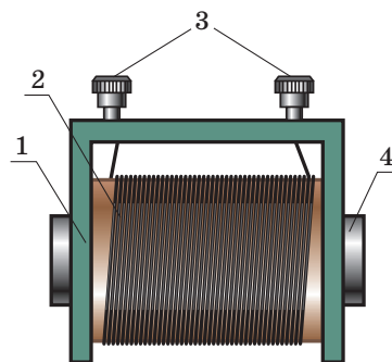
Рис. 6.2. Будова електромагніта: 1 — каркас; 2 — обмотка; 3 — клемми; 4 — осердя
