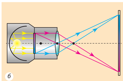
Рис. 15.4. а — побудова зображення A_1B_1 предмета AB у збиральній лінзі: предмет AB розташований між фокусом і подвійним фокусом лінзи; б — хід променів у проєкційному апараті
