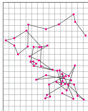
Рис. 40.3. Копія малюнка французького фізика Жана Батиста Перрена (1870–1942), на якому відтворено результати спостереження в мікроскоп броунівської частинки — дрібної частинки речовини, завислої в рідині. Броунівський рух частинок, викликаний хаотичними ударами по них молекул, підтверджує атомарну будову матерії
