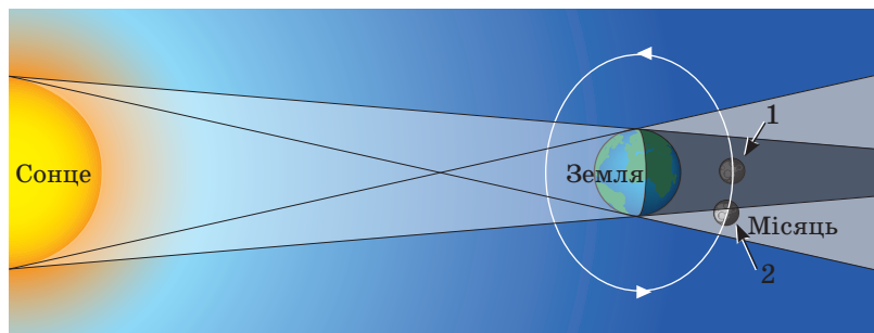
Рис. 10.8. Місячне затемнення: а — повне (Місяць у положенні 1); б — часткове (Місяць у положенні 2)
