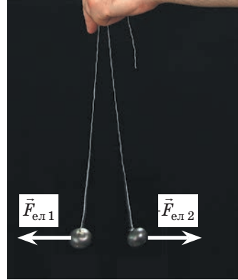
Рис. 32.4. На кожну з двох од- нойменно заряджених кульок діє сила Кулона з боку іншої кульки. Ці сили є рівними за модулем і протилежними за напрямком: \vec{F}_{\text{ел}1} = -\vec{F}_{\text{ел}2}
