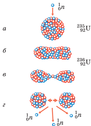
Рис. 26.1. Схема поділу ядра Урану. Поглинаючи нейтрон (а), ядро Урану збуджується й набуває видовженої форми (б); поступово розтягуючись (в), нове нестійке ядро розпадається на два осколки (г)
