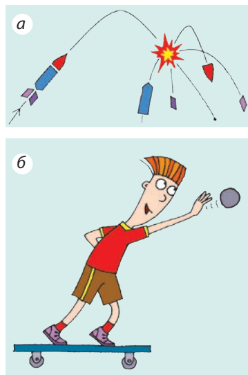
Рис. 36.1. Якщо зовнішні сили, що діють на систему, зрівноважені або значно менші від внутрішніх сил системи, цю систему можна вважати замкнутою
