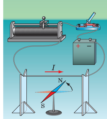
Рис. 1.1. Схема досліді Ерстеда (Тут і далі наявність символу I означає, що в провіднику тече струм; стрілка поряд показує напрямок струму.)
