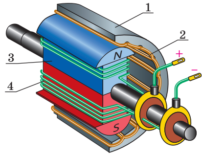
Рис. 8.7. Схема будови електромеханічного генератора:
