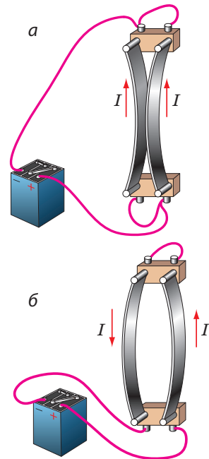
Рис. 1.2. Схема досліді А. Ампера. Якщо у двох паралельних провідниках течуть струми одного напрямку, провідники притягуються (а); якщо течуть струми протилежних напрямків, провідники відштовхуються (б)
