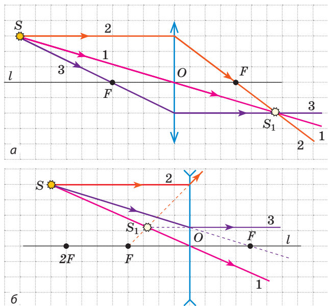
Рис. 15.2. Три найпростіші в побудові промені («зручні промені»): 1 — промінь, який проходить через оптичний центр O лінзи, — не заломлюється та не змінює свого напрямку; 2 — промінь, паралельний головній оптичній осі l лінзи, — після заломлення в лінзі йде через фокус F (а) або через фокус F йде його продовження (б); 3 — промінь, який проходить через фокус F , — після заломлення в лінзі йде паралельно головній оптичній осі l лінзи (а, б)
