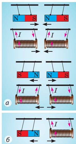
Рис. 1.3. Катушки зі струмом поводяться як постійні магніти
