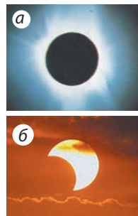
Рис. 10.7. Сонячне затемнення: а — повне (в області повної тіні); б — часткове (в області півтіні)
