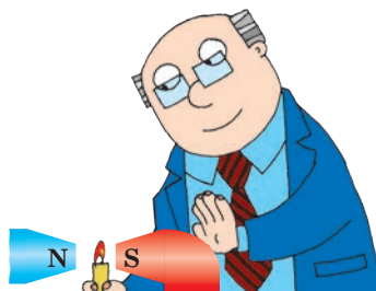
Рис. 5.3. Полум'я свічки виштовхується з магнітного поля, оскільки продукти згоряння є діамагнітними частинками
