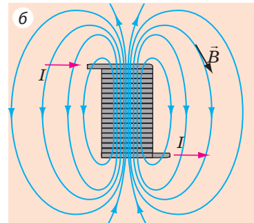
Рис. 3.6. Лінії магнітної індукції магнітного поля штабового магніту (а) і котушки зі струмом (б)
