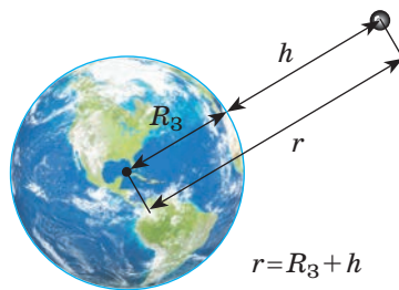
Рис. 33.6. Відстань r від центра Землі до тіла дорівнює сумі радіуса Землі R_3 і висоти h , на якій перебуває тіло
