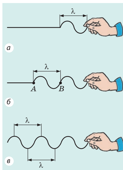
Рис. 17.8. Довжина хвилі дорівнює відстані, на яку поширюється хвиля за час одного коливання (це також відстань між двома найближчими гребнями або між двома найближчими западинами)
