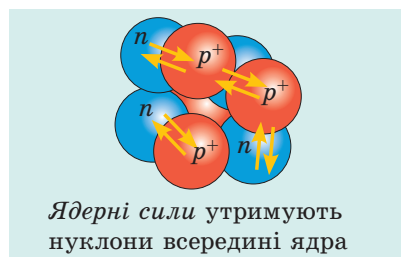
Рис. 22.8. Сили взаємодії між нуклонами ядра
