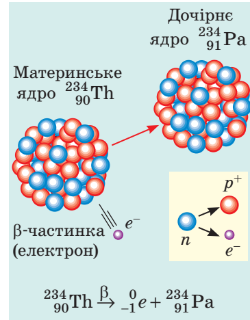
Рис. 23.8. Під час \beta -розпаду один із нейтронів материнського ядра перетворюється на протон і електрон; електрон випромінюється, а протон залишається в ядрі (утворюється нове ядро)
