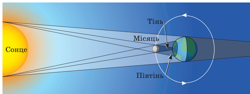
Рис. 10.7. Сонячне затемнення: а — повне (в області повної тіні); б — часткове (в області півтіні)
