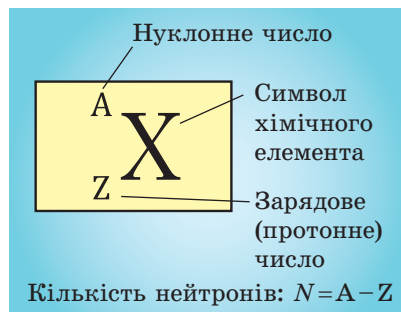
Рис. 22.6. Позначення нукліда хімічного елемента
