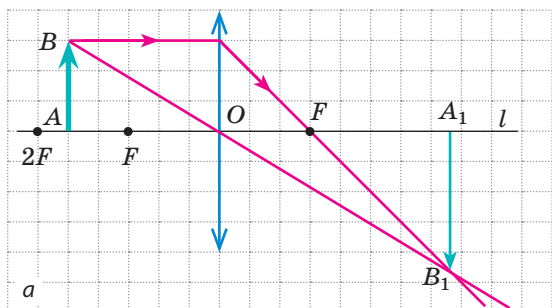
Рис. 15.4. а — побудова зображення A_1B_1 предмета AB у збиральній лінзі: предмет AB розташований між фокусом і подвійним фокусом лінзи; б — хід променів у проєкційному апараті
