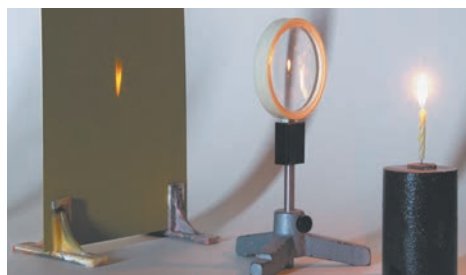
Рис. 15.1. Отримання зображення полум'я свічки за допомогою збиральної лінзи
