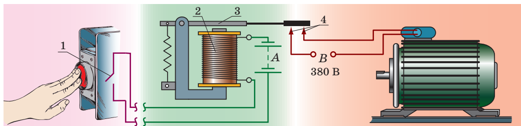
Рис. 6.6. Принцип дії електромагнітного реле. Коли замикають ключ (1) (натискають кнопку), в обмотці електромагніта (2) йде слабкий безпечний струм. Унаслідок цього залізне осердя електромагніта притягує до себе якір (3). Коли якір опускається і замикає контакти (4), замикається коло електродвигуна, який споживає струм значно більшої сили
