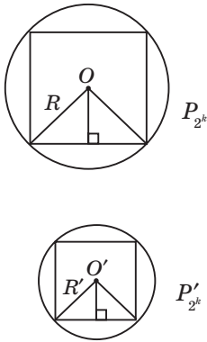
Рис. 159. До обґрунтування формули довжини кола
