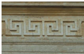
Меандр
