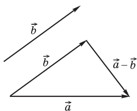
Рис. 100. Побудова різниці векторів
