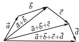
Рис. 99. Побудова суми векторів за правилом многокутника
