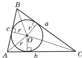
Рис. 23. До доведення формули радіуса вписаного кола
