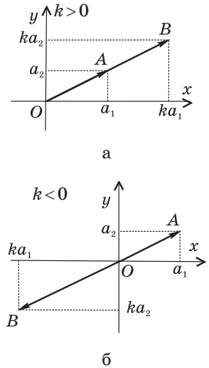
Рис. 107. Побудова вектора ka
