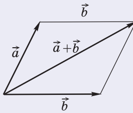
Правило паралелограма
