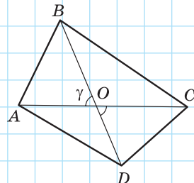
Рис. 22. До доведення формули площі чотирикутника
