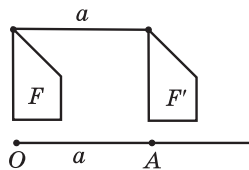
Рис. 64. Паралельне перенесення фігури F у напрямі променя OA на відстань a
