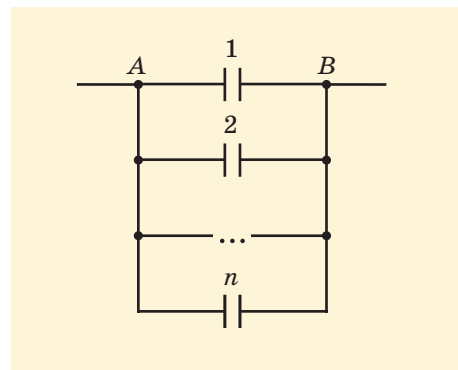
Рис. 33.9. Паралельне з'єднання конденсаторів
