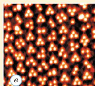
Рис. 20.3. Отримані за допомогою різних приладів зображення структури речовини: а — зображення вольфрамового вістря в йонному проекторі; б — зображення поверхні кристала ніобію, отримане за допомогою електронного мікроскопа і збільшене в 6 млн разів; в — зображення поверхні кристала германію, отримане за допомогою скануючого тунельного мікроскопа
