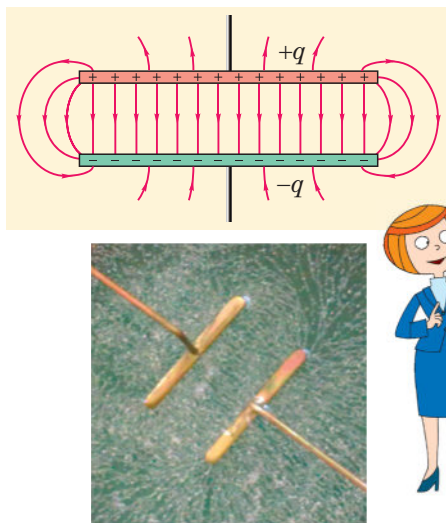
Рис. 33.6. Силкові лінії електричного поля плоского конденсатора (поблизу країв конденсатора його поле є неоднорідним; існує також слабе поле поза конденсатором)
