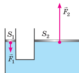
Рис. 14.2. Гідравлічна машина
