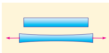
Рис. 27.4. Під час розтягнення змінюються й поперечні розміри стрижня
