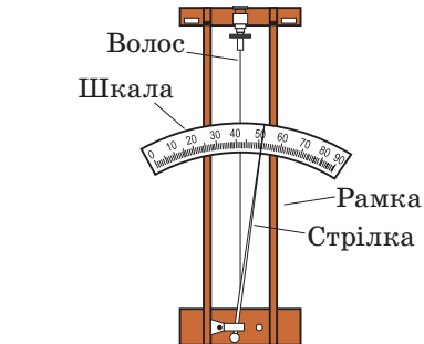
Рис. 24.6. Гігрометр волосяний
