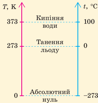
Рис. 22.5. Температурні шкали Цельсія та Кельвіна (зазначені температури відповідають таненню льоду та кипінню води за нормального атмосферного тиску)
