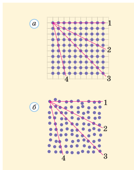
Рис. 27.1. До ілюстрації причин анізотропії кристалів. Схематичне зображення структури: а — кристала; б — речовини без дальнього порядку
