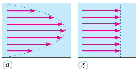
Рис. 14.5. Червоними стрілками показано швидкості ламінарного руху різних шарів рідини в трубі: а — реальна картина; б — спрощена модель без урахування в'язкості
