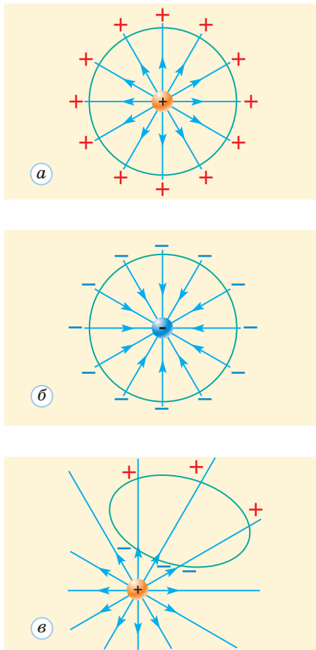
Рис. 30.16. Тільки «внутрішні» заряди створюють потік \vec{E} через замкнену поверхню
