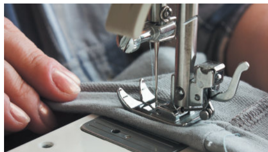
Рис. 16.10. Приклади вимушених коливань
