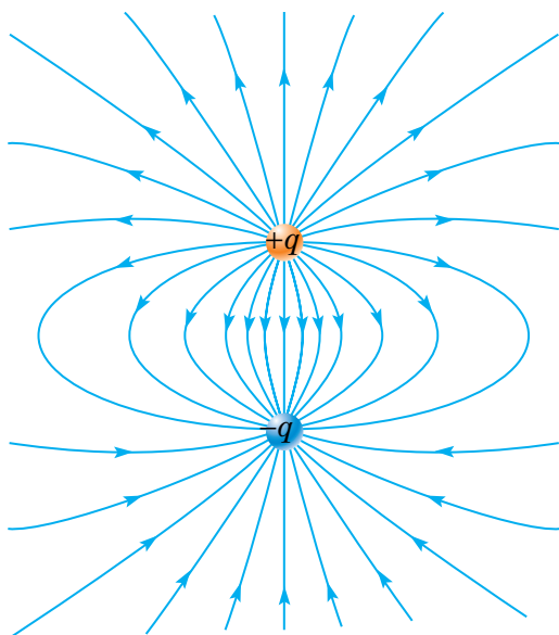
Рис. 30.12. Силкові лінії електричного поля диполя
