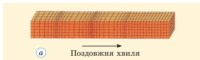
Рис. 17.3. Схематичне зображення поздовжніх (а) і поперечних (б) хвиль у твердому тілі
