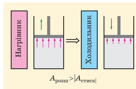
Рис. 29.3. Проста модель теплового двигуна: завдяки використанню холодильника під час стискання газу витрачають менше енергії, ніж отримують під час розширення
