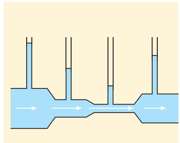
Рис. 14.9. Порівняння тиску в різних ділянках труби. Білими стрілками показано швидкості руху рідини на різних ділянках труби
