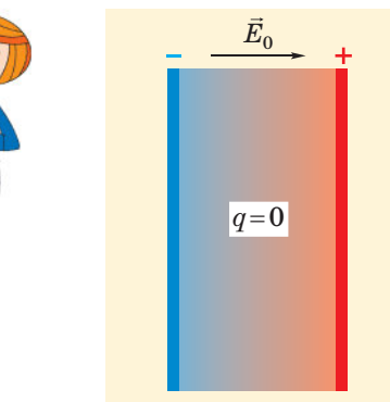
Рис. 31.6. Поляризація діелектричної пластини під дією електричного поля: на поверхнях виникають зв'язані заряди протилежних знаків
