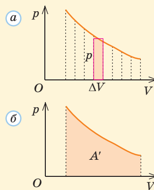
Рис. 28.3. Знаходимо роботу газу під час довільного процесу: а — площа прямокутної смужки дорівнює площі зафарбованої ділянки під графіком; б — сумарна площа всіх таких смужок чисельно дорівнює роботі газу A'
