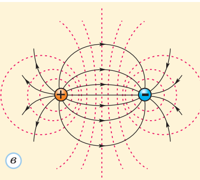
Рис. 32.5. Еквіпотенціальні поверхні (червоні штрихові лінії) перпендикулярні до силових ліній. Різниця потенціалів для всіх сусідніх еквіпотенціальних поверхонь однакова
