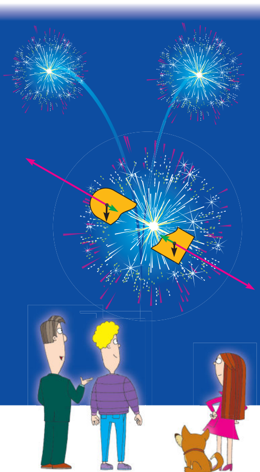
Рис. 13.1. Розрив спеціального снаряда під час феєрверка. Для двох осколків показано діючі сили: червоним — сили тиску порохових газів (внутрішні сили в системі); чорним — сили тяжіння; зеленим — сили опору повітря
