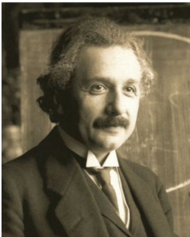
Рис. 18.1. Альберт Ейнштейн (1879–1955) — один із творців сучасної фізики. Створив спеціальну теорію відносності, теорію тяжіння (загальну теорію відносності), теорію фотоелефекту. Передбачив існування вимушеного випромінювання (на якому ґрунтується дія лазера), розвинув статистичну теорію броунівського руху, створив квантову статистику частинок із цілим спіном. Лауреат Нобелівської премії з фізики (1921), великої кількості нагород від академій практично всіх країн світу. 2005 рік був оголошений ЮНЕСКО роком фізики саме з нагоди століття відкриття спеціальної теорії відносності Альбертом Ейнштейном
