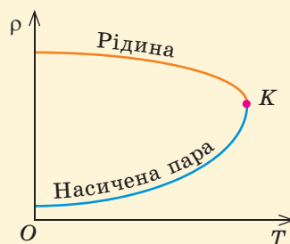
Рис. 25.2. Графіки (схематичні, без додержання масштабу) залежності густини рідини та її насиченої пари від температури. Точка K відповідає критичному стану
