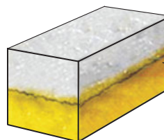
Рис. 20.4. Дифузія свинцю та золота поступово спричиняє «зростання» двох брусків із різних металів, тобто їх взаємне проникнення та утворення на межі шару «сплаву»
