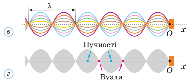
Рис. 17.10. Утворення стоячої хвилі: а — хвиля біжить до закріпленого кінця шнура; б — відбита хвиля; в — результат накладання двох хвиль — стояча хвиля; г — видимі розміти контури шнура
