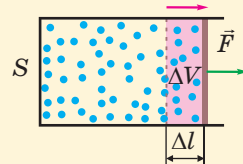
Рис. 28.2. Виводимо формулу для роботи газу під час ізобарного процесу
