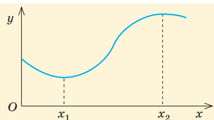
Рис. 5. Зв'язок похідної функції зі зростанням і убыванням цієї функції: y'(x) < 0 на інтервалі 0 < x < x_1 ; y'(x) > 0 на інтервалі x_1 < x < x_2 . У точках мінімуму x_1 та максимуму x_2 похідна функції дорівнює нулю
