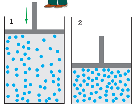
Рис. 23.1. Повільне стискання газу відбувається за незмінної температури. При цьому збільшується концентрація молекул і кількість їх зіткнень з поршнем і стінками, які відбуваються щосекунди
