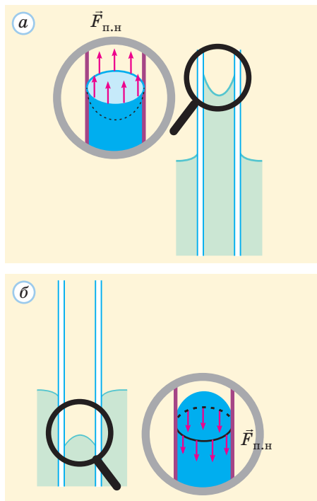
Рис. 26.5. Рівновага рідини у вертикальному циліндричному капілярі у випадку: a — змочування; б — незмочування
