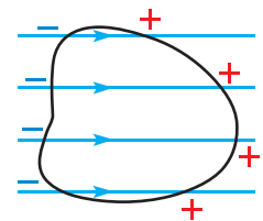
Рис. 30.15. Кількість силових ліній, що перетинають поверхню, пропорційна \cos \alpha та модулю напруженості електричного поля; для замкненої поверхні лінії, що входять усередину, слід «рахувати» зі знаком мінус
