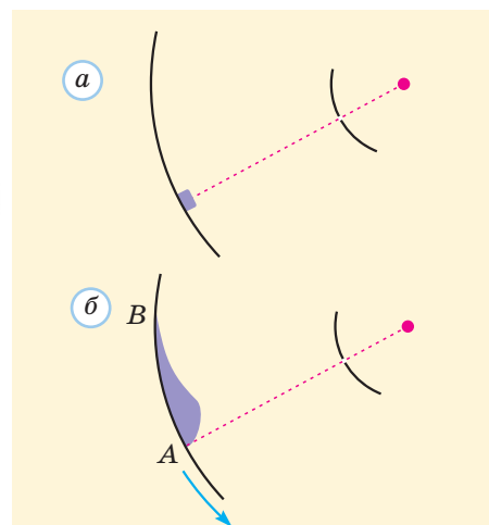
Рис. 22.7. Профіль смужки срібла в досліді Штерна: а — за нерухомого приладу; б — за умови його обертання. Поблизу точки А розмітої смужки осідають атоми з найбільшими швидкостями, поблизу точки В — з найменшими
