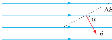
Рис. 30.15. Кількість силових ліній, що перетинають поверхню, пропорційна \cos \alpha та модулю напруженості електричного поля; для замкненої поверхні лінії, що входять усередину, слід «рахувати» зі знаком мінус
