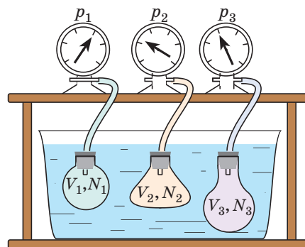
Рис. 22.4. Експеримент, що дозволяє перевірити зв'язок між температурою газу та середньою кінетичною енергією поступального руху його молекул
