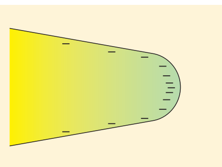
Рис. 31.2. Неоднорідний розподіл електричних зарядів по поверхні провідника біля вістря
