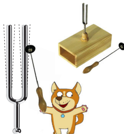
Рис. 17.12. Камертон
