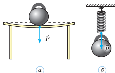
Рис. 7.3. Вага тіл, що мають опору або підвіс
