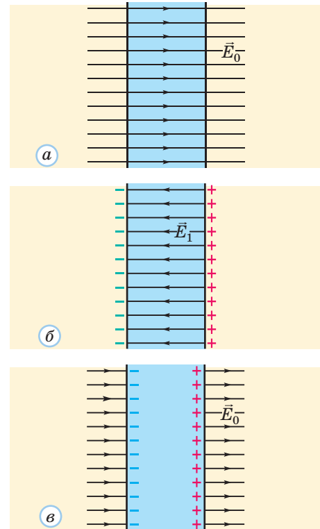
Рис. 31.1. У провіднику під дією зовнішнього електричного поля з напруженістю \vec{E}_0 відбувається перерозподіл зарядів; ці заряди створюють усередині провідника власне електричне поле з напруженістю \vec{E}_1 = -\vec{E}_0 , яке компенсує зовнішнє поле
