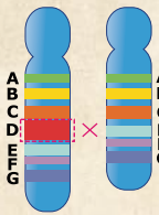
Делеція
