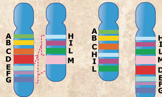
Транслокація
