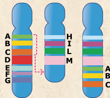
Інсерція
