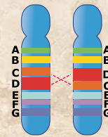
Інверсія
