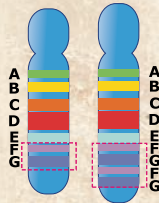
Дуплікація
