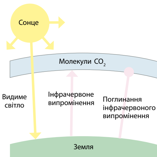
Мал. 37.3. Механізм затримання енергії парниковими газами
