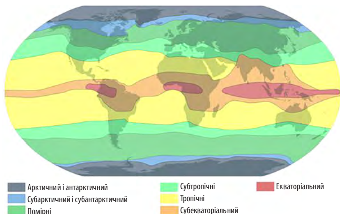
Мал. 2. Картохема кліматичних поясів за Б. Алісовим.
