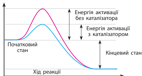
Мал. 38.2. За умови ферментативного каталізу знижується енергія активації реакції
