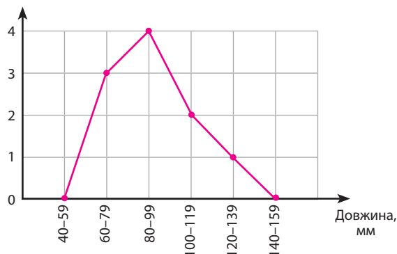
Мал. 67.4. Варіаційна крива довжини листків
