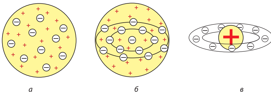
Мал. 6.1. а — «кексова» модель атома Вільяма Томсона (1902), який уявляв атом як згусток позитивно зарядженої матерії, де рівномірно розподілені електрони, наче родзинки в кексі; б — «кексова» модель, удосконалена Джозефом Джоном Томпсоном (1904), у якій електрони розміщені в одній площині й утворюють концентричні кільця; в — модель атома Хантаро Нагаока (1904), який припустив, що атом схожий на планету Сатурн: половину об'єму займає позитивно заряджена куля, навколо якої супутники-електрони утворюють кільце
