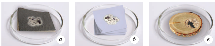
Мал. 31.5. Луги — надзвичайно їдкі речовини: а — луг перетворює тканину на драглеподібну масу; б — луг утворює дірки в папері; в — луг пошкоджує деревину
