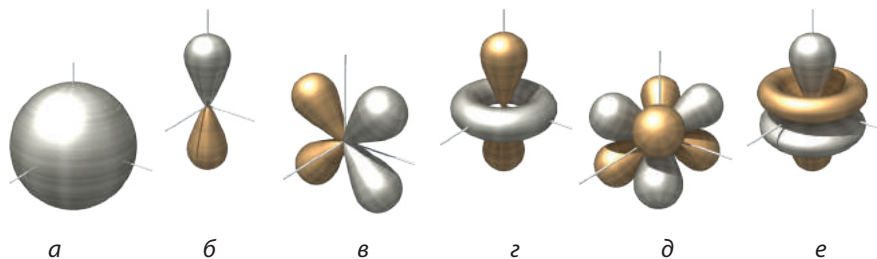
Мал. 8.3. Атомні орбіталі: а — s -орбіталь; б — p -орбіталь; в і г — різні види d -орбіталей; д і е — різні види f -орбіталей
