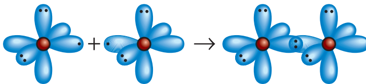
Мал. 18.2. Перекривання p -орбіталей атомів Флуору під час утворення молекули фтору. Інші p -орбіталі, на яких перебувають електронні пари, не беруть участі в утворенні зв'язку
