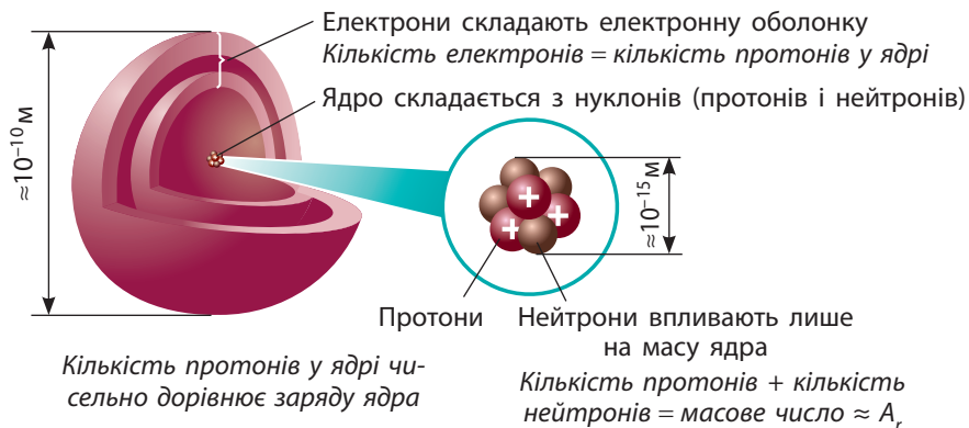
Мал. 6.5. Склад атома
