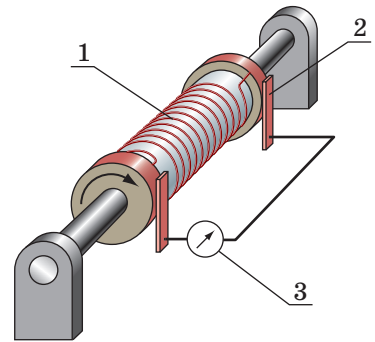
Рис. 36.2. Схема пристрою для вивчення природи електричного струму в металах: 1 — котушка з металевим дротом; 2 — ковзні контакти; 3 — чутливий гальванометр. Котушці надають швидкого обертання й різко зупиняють. У результаті в колі виникає електричний струм, який реєструється гальванометром
