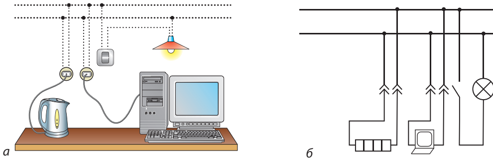
Рис. 32.5. Частина електричної проводки у квартирі: а — загальний вигляд; б — схематичне зображення. На практиці електропроводку монтують у стінах
