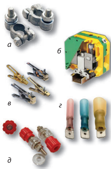
Рис. 26.2. Різні затискачі (клемми) для з'єднування провідників: акумуляторні (а); високовольтні (б); заземлення (в); ножові (г); приладні (д)
