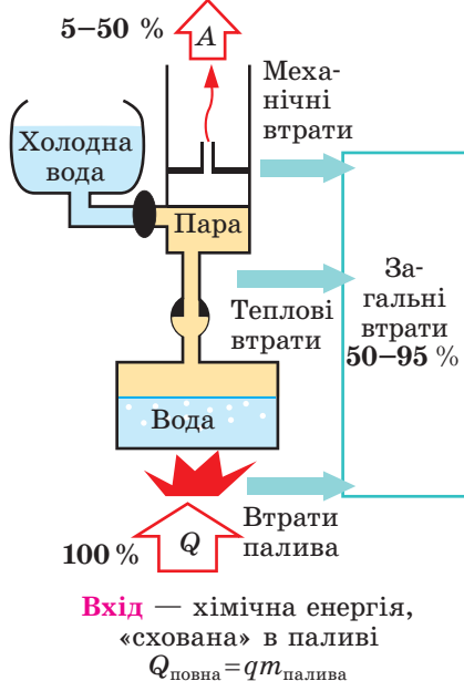
Рис. 16.3. ККД парових теплових двигунів і схема втрат енергії
