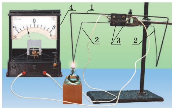
Рис. 25.4. Термопара — пристрій для перетворення теплової енергії на електричну. До кінців константового дроту (1) припаяно два залізні дроти (2), вільні кінці яких (3) з'єднані з гальванометром* (4). Якщо нагріти місце спаю, гальванометр зафіксує наявність струму
