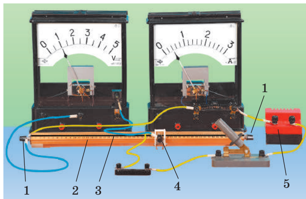
Рис. 30.1. Дослід, який доводить, що опір провідника прямо пропорційний його довжині. На рисунку: 1 — клемми; 2 — лінійка; 3 — ніхромовий дріт (провідник); 4 — повзунок; 5 — джерело струму
