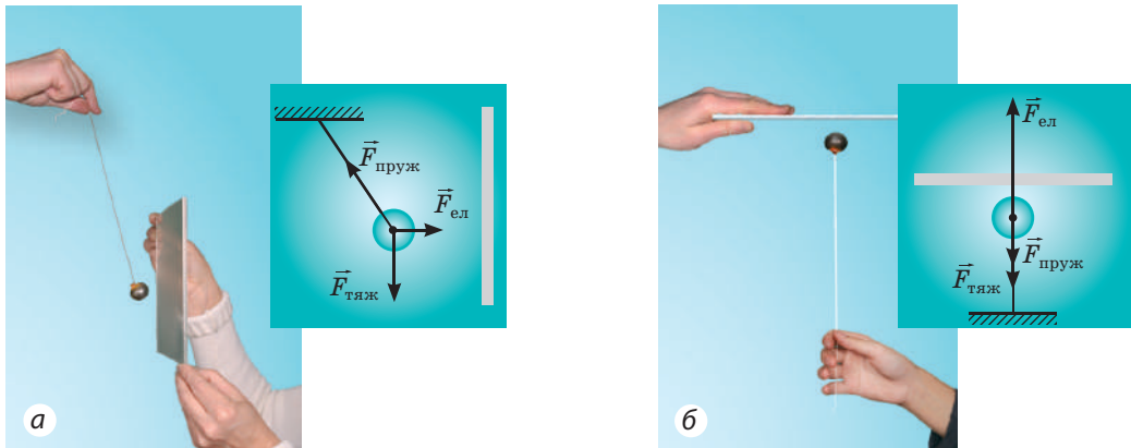
Рис. 20.1. Негативно заряджена кулька притягується до позитивно зарядженої пластини з оргскла. Кулька перебуватиме в спокої, коли сила тяжіння \vec{F}_{\text{тяж}} і сила натягу нитки \vec{F}_{\text{нат}} будуть скомпенсовані силою \vec{F}_{\text{ел}} , яка діє на кульку з боку наелектризованої пластини
