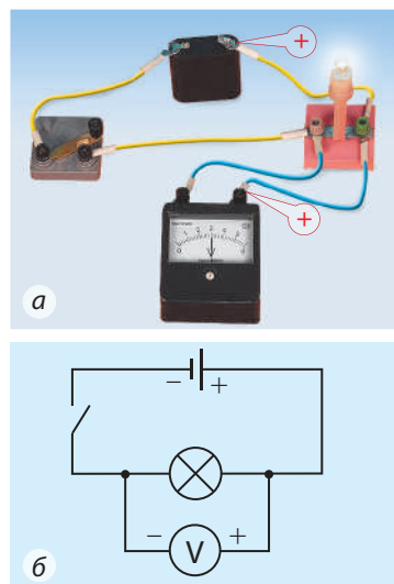
Рис. 28.2. Вимірювання вольтметром напруги на лампі: а — загальний вигляд; б — схема електричного кола
