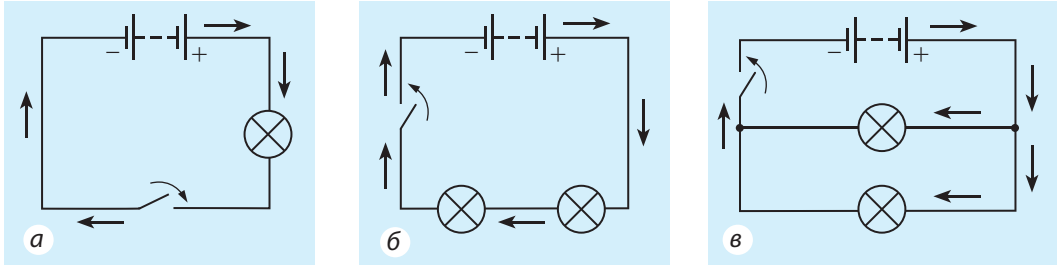
Рис. 26.5. Схеми деяких електричних кіл: а — схема електричного кола вмикання лампи (див. рис. 26.1 ); б — схема послідовного з'єднання двох ламп (див. рис. 26.3, а ); в — схема паралельного з'єднання двох ламп (див. рис. 26.3, б ). Стрілками позначено напрямки струму в разі замкнення ключа
