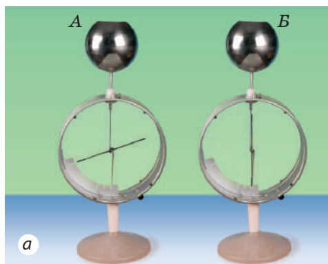
Рис. 23.1. Якщо заряджений електрометр з'єднати з незарядженим за допомогою провідника, частина заряду перейде на незаряджений електрометр
