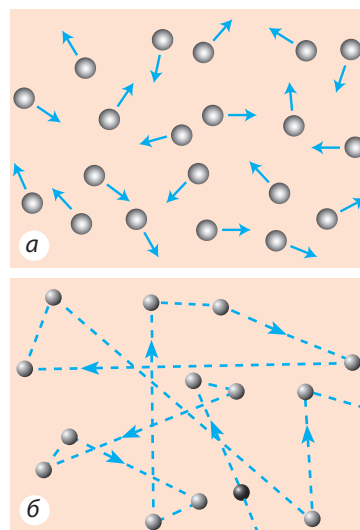
Рис. 10.7. Рух і розташування частинок газу: а — напрямки руху частинок змінюється в результаті зіткнення з іншими частинками; б — приблизна траєкторія руху частинки (збільшено в мільйон разів)
