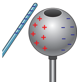
Рис. 21.4. Унаслідок дії електричного поля негативно зарядженої палички ближча до неї частина металевої сфери набуває позитивного заряду
